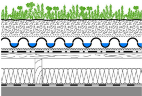
Abb. 26 Schnitt Kaltdach (BuGG)
