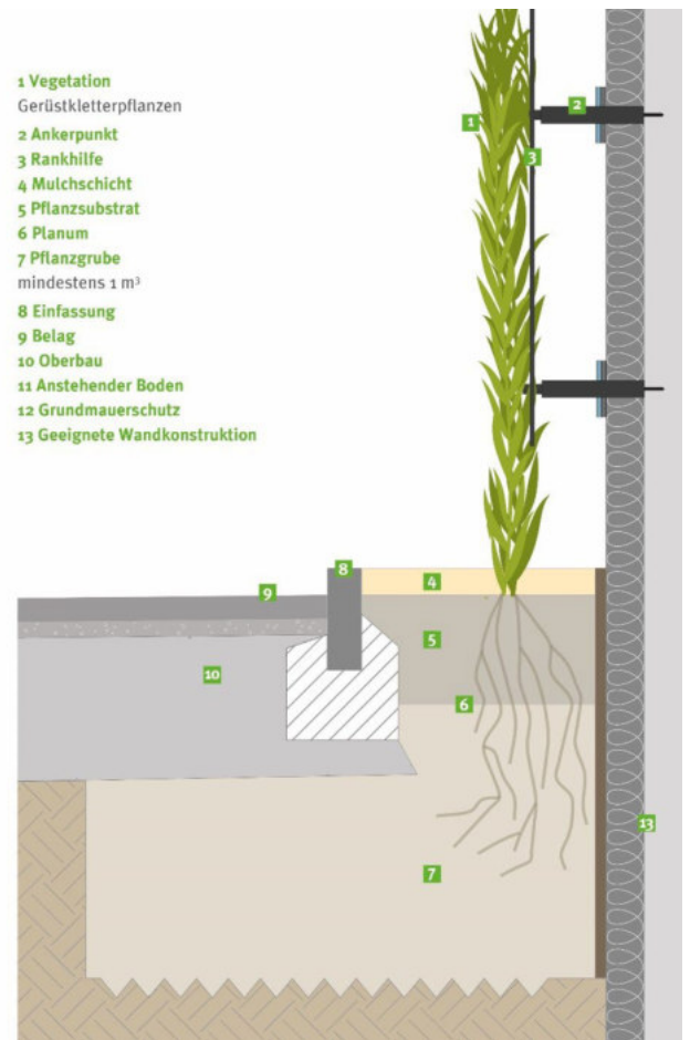
Abb. 34 Schnitt bodengebundene Fassadenbegrünung mit Kletterhilfe (BuGG)
