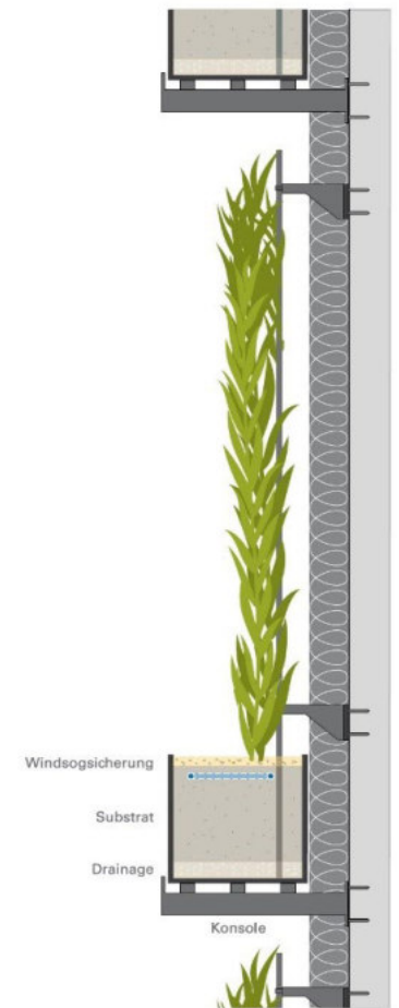
Abb. 43 Schnitt wandgebundene Fassadenbegrünung in Regalbauweise (BuGG)
