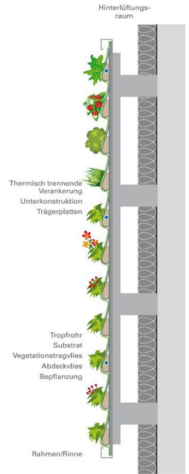
Abb. 39 Schnitt wandgebundene Fassadenbegrünung mit Vlies (BuGG)
