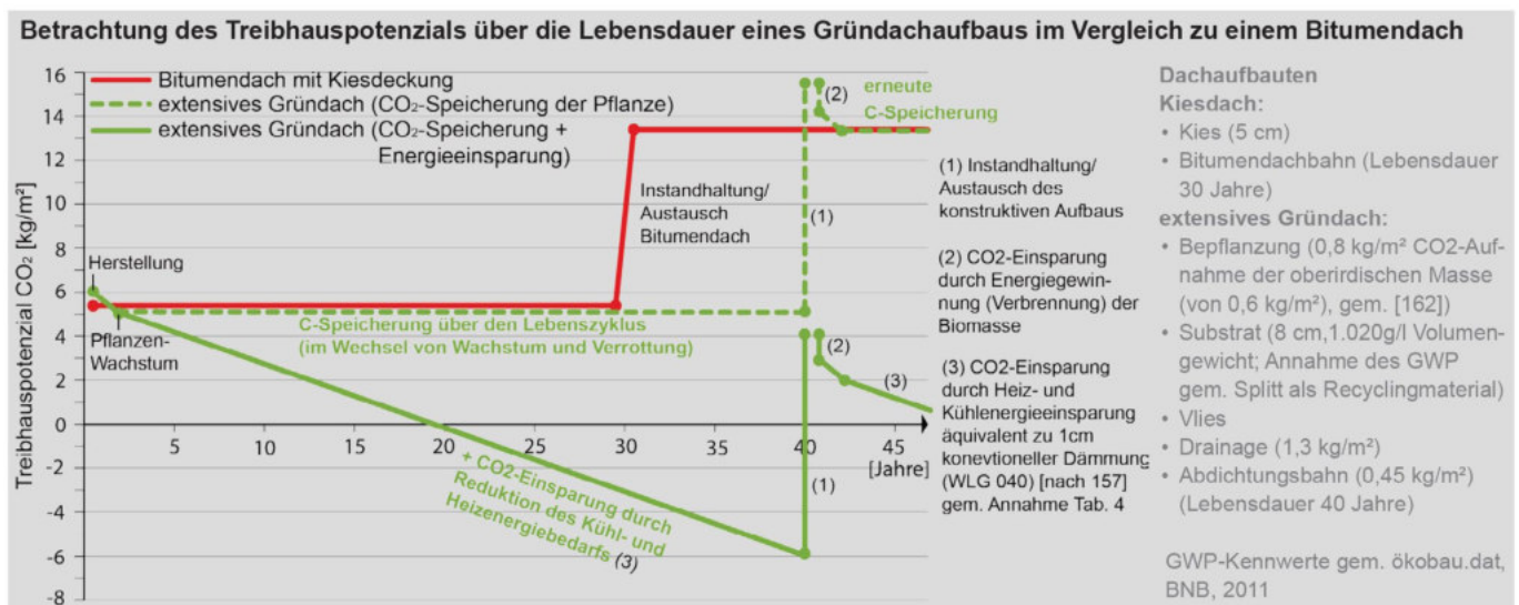
Abb. 57 Betrachtung des Treibhauspotenzials über die Lebensdauer eines Gründachaufbaus im Vergleich zu einem Bitumendach (Pfooser et al 2013)
