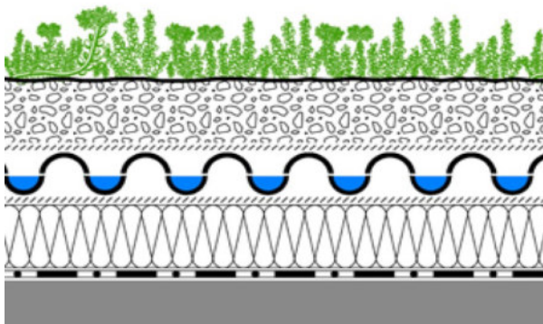
Abb. 25 Schnitt Umkehrdach (BuGG)
