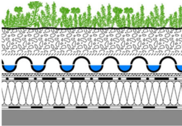
Abb. 24 Schnitt Warmdach (BuGG)
